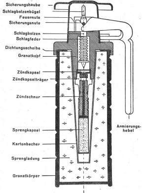
Die schweizerische Defensiv-Handgranate Modell 1917 und deren Längsschnitt. (A Er 0219.) La grenade à main défensive suisse, modèle 1917, et sa coupe en long. La granata a mano difensiva, modello 1917 possiede un corpo di ghisa dipinto in giallo e grigio. Agisce per lo scoppio delle sue robuste pareti entro un raggio di ben 50 metri. Pesa quasi il doppio della granata offensiva.
