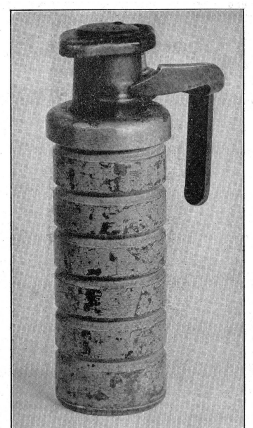
Die schweizerische Defensiv-Handgranate Modell 1917 und deren Längsschnitt. (A Er 0219.) La grenade à main défensive suisse, modèle 1917, et sa coupe en long. La granata a mano difensiva, modello 1917 possiede un corpo di ghisa dipinto in giallo e grigio. Agisce per lo scoppio delle sue robuste pareti entro un raggio di ben 50 metri. Pesa quasi il doppio della granata offensiva.
