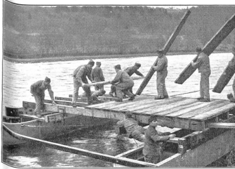
Wann sind die Tragbalken fixiert, so schiff auch schon der Ladestrupp die massiven Bodenbretter heran. (A Er 0308.)
