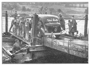
Die Drahtseilgeländer sind noch nicht gestreckt, als der erste Wagen zum Uebersetzen auf die Fähre dirigiert wird. Knapp 45 Minuten dauerte der Einbau der Fähre. (A Er 0305.)
