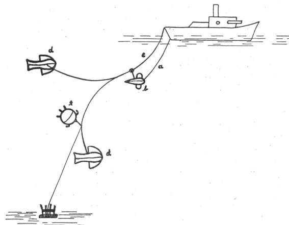
rätes maßgebende Otter (b) an der Tiefenleine (a) nachgeschleppt; die glatten Räumleinen (c) laufen vom Schiffsheck durch die Führungsrolle der Tiefenotter (b) zu den beiden Seitenottern (d). Das von der Räumleine
