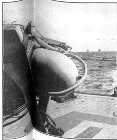
Bild 2: Links: Minenwurf aus einem englischen Minenleger. Die Geleise der Lagerräume enden in den Abwurfseilen, über welche die Minen in genau bestimmten Zeitabständen in das Wasser gestoßen werden.
