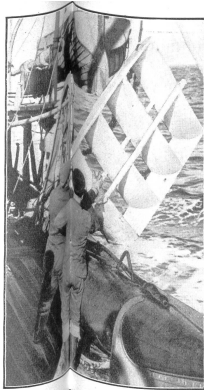
Bild 4: Links: Auswerfen des Drahtens eines Einschiff-Minensuchgerätes, durch welchen das Gerät auf die gewünschte Tiefe gesteuert wird.
