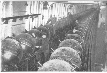
Bild 1: Minenlagerraum im englischen Minenkreuzer «Adventure», welcher ein Fassungsvermögen von 340 Minen besitzt. Die Minen ruhen auf den am Ankerkasten fixierten Laufrädern direkt in Geleisen, welche zu den Abwurfstellen am Hinterschiff führen.
