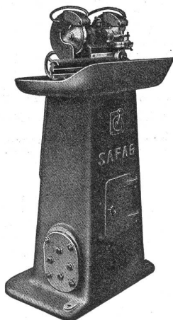
Maschine zum Schleifen von Hartmetallrehstählen
