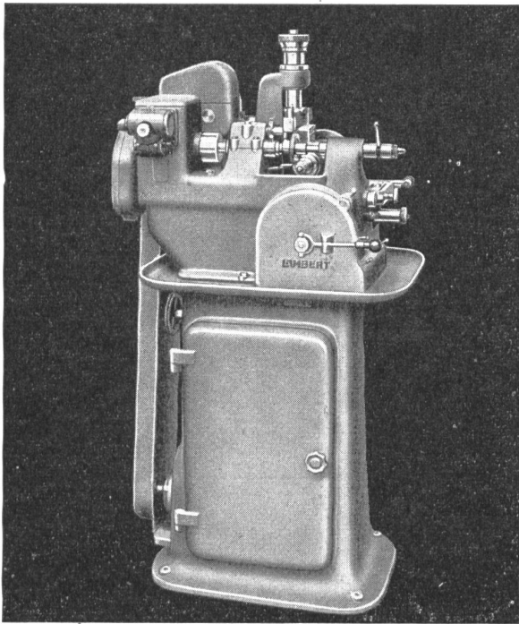
Abwälzräderfräsmaschine Type 75
