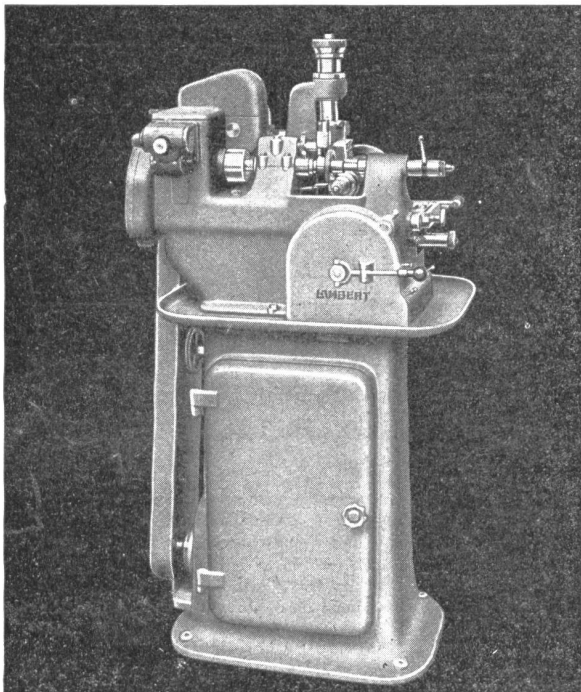
Abwälräderfräsmaschine Type 75
