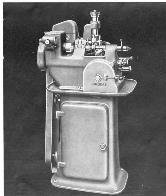
Abwälzräderfrasmachine Type 75
