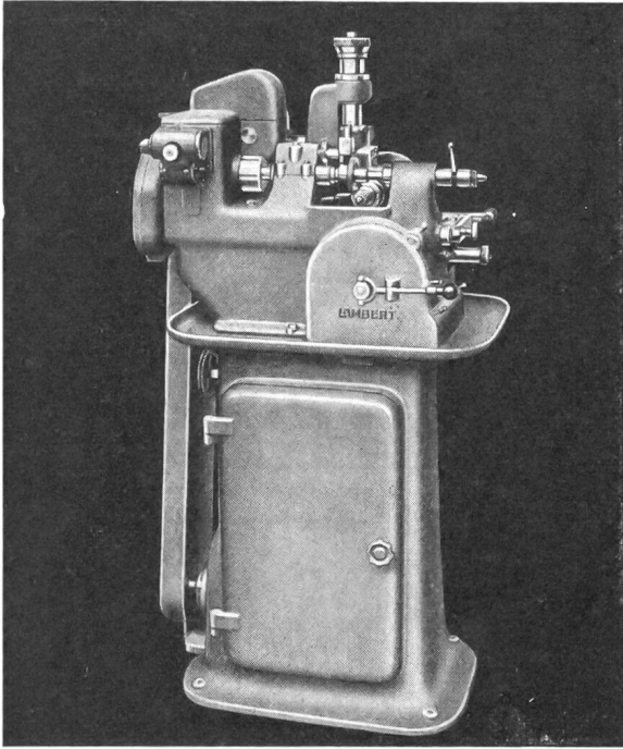
Abwälzräderfräsmaschine Type 75
