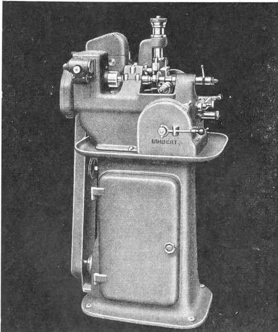
Abwälzräderfräsmaschine Type 75
