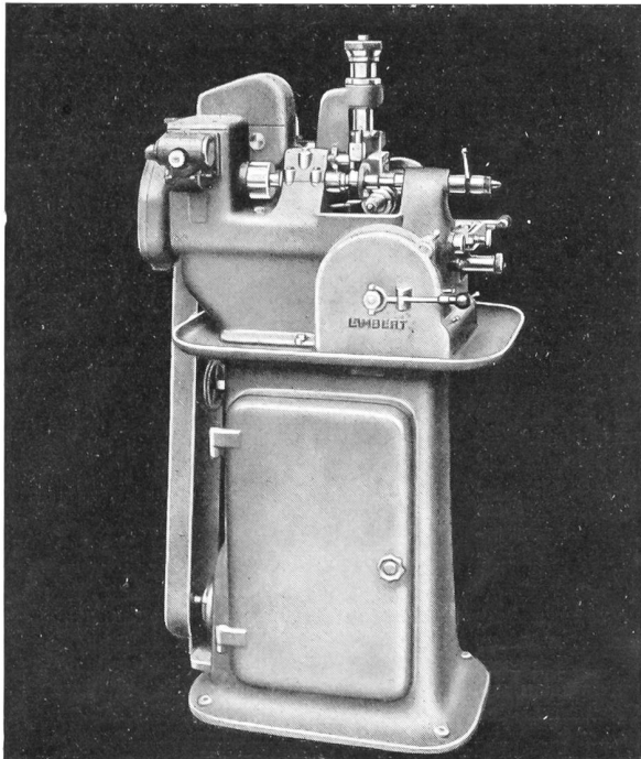
Abwälzräderfräsmaschine Type 75
