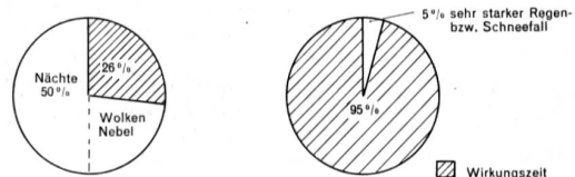
Optisch gesteuerte Batterie — Radargesteuerte Batterie
