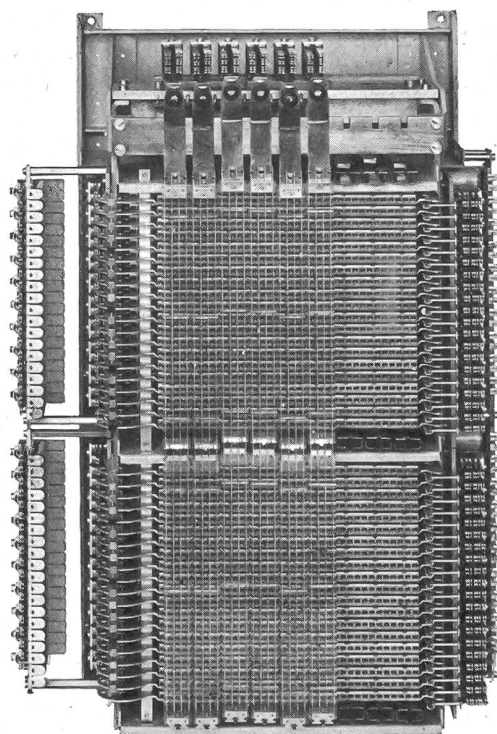
Der Kreuzwähler Gfeller zur Verwendung in der automatischen Telephonie
