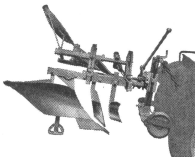
Anbaukultivator
