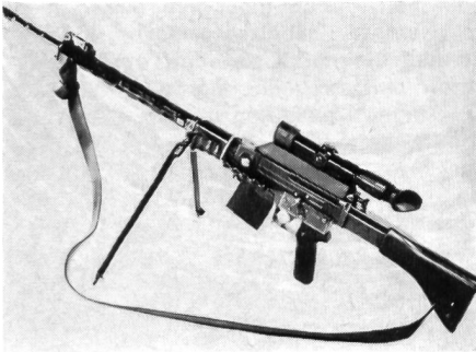
Eine neue Zielvorrichtung für das Armee-Sturmgewehr
