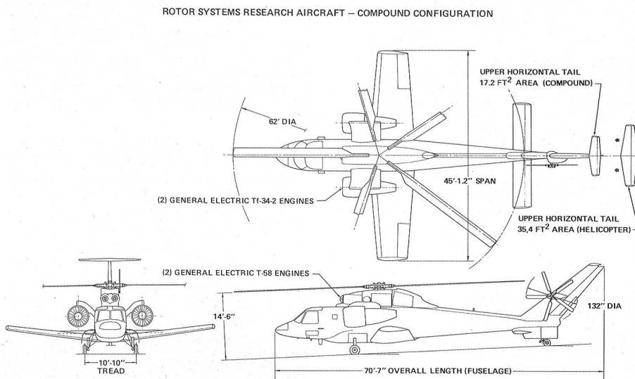
SIKORSKY S-72
