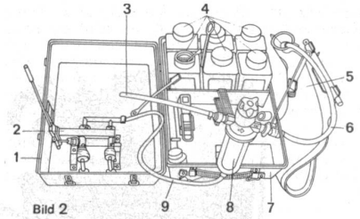
Bild 2 Skizze der einsatzbereiten WFS 1
