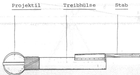
Bild 15 Die drei Hauptteile der Kriegsrakete.
