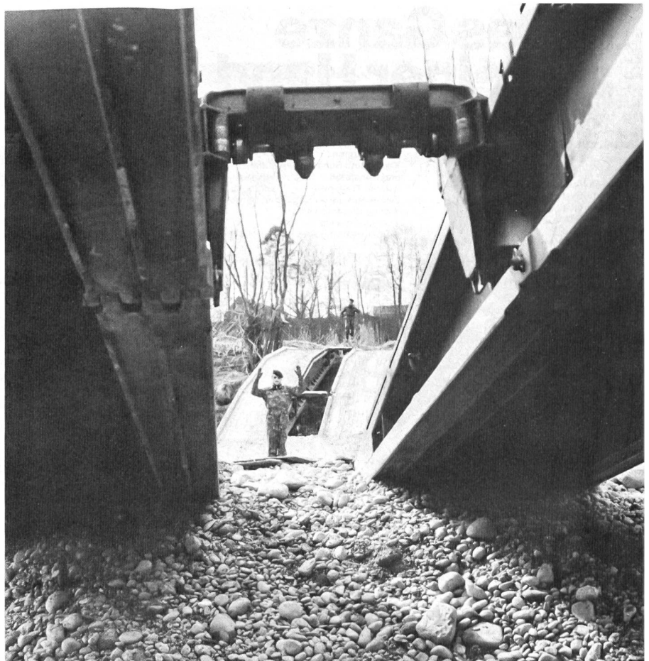
Einsatz Brückenlegepanzer
