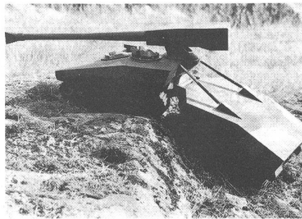
Wie gelenkig der Prototyp des Kampffahrzeugs ist, beweist die mühevolle Geländefahrt über Stock und Stein.
