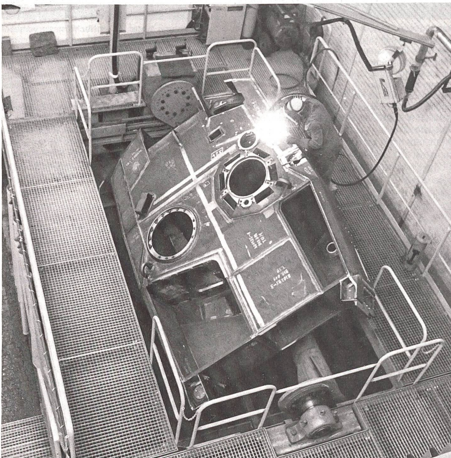
Die Fertigung des Roh-Turmgehäuses erfordert anspruchsvolle Schweiss-, Füge- und Prüfarbeiten durch ausgebildete Fachleute.
