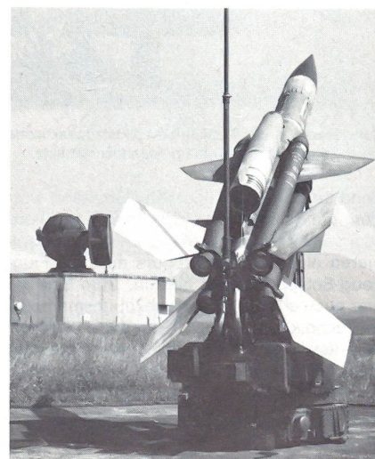
Bloodhound BL-64 Lenkwaffenstellung mit Radareinheit.
