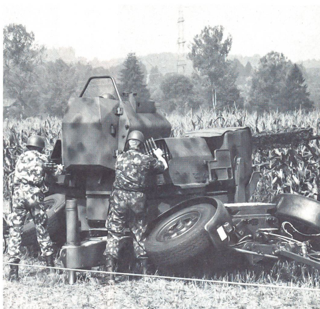
Aufmunitionieren der Nachladeautomaten der 35mm Flab Kan 63/90.
