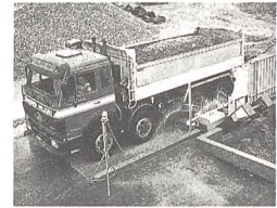
MOBY DICK Reifenwaschanlagen und Radreinigungsanlagen für LKWs
