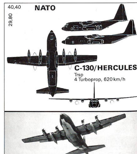
C-130 Hercules
