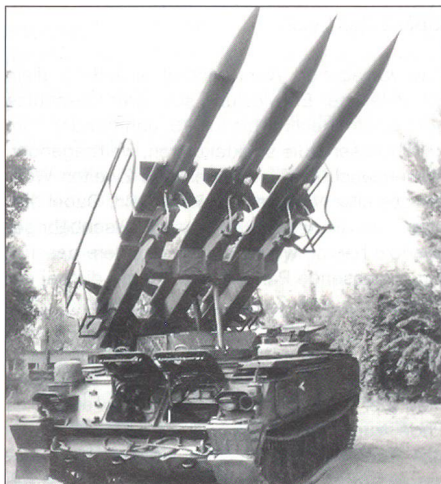
Fliegerabwehrenkennungswaffe GM578 SzPU «KUB» (SA-6) der ungarischen Streitkräfte.
