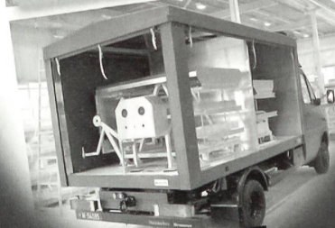
FHS-Spezial-Wechselaufbau
