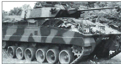
Warrior mit neuem CTA-Turm und 40-mm-Kanone.
