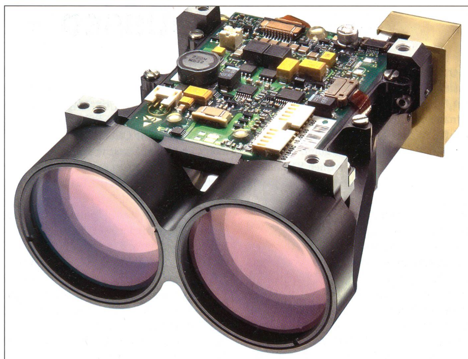
Welche technologische Komplexität ein Sensor heute aufweist zeigt das Bild mit den Innereien eines derartigen Systems.
