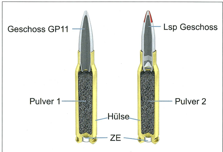
Der Aufbau der GP-11-Patrone.
