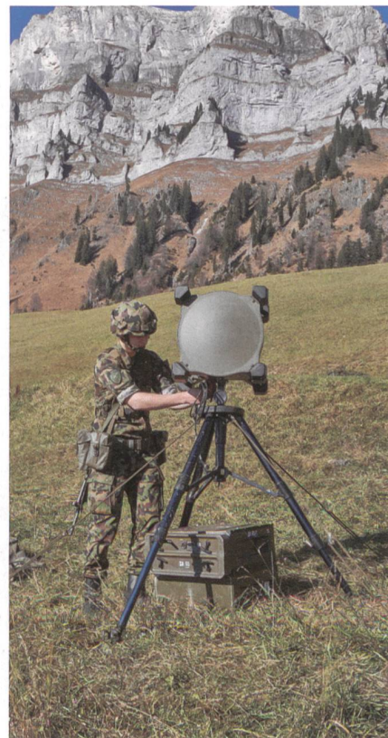
Das statisch eingesetzte Richtstrahlssystem R-905 der Schweizer Armee mit hoher Autonomie und Datendurchsatz.
