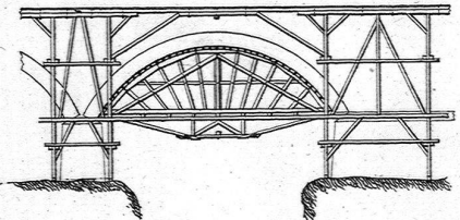
Gewölberüste Forderansicht
