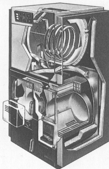
Hoval DuoLyf Niedertemperatur- Doppelkessel mit aufgebautem, vom Kessel getrennten Boiler
