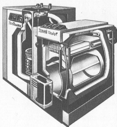
Hoval UnoLyf Niedertemperatur- Öl-/Gaskessel mit Beistellboiler Hoval CombiVal
