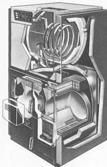
Hoval DuoLyt Niedertemperatur- Doppelkessel mit aufbautem, vom Kessel getrennten Boiler
