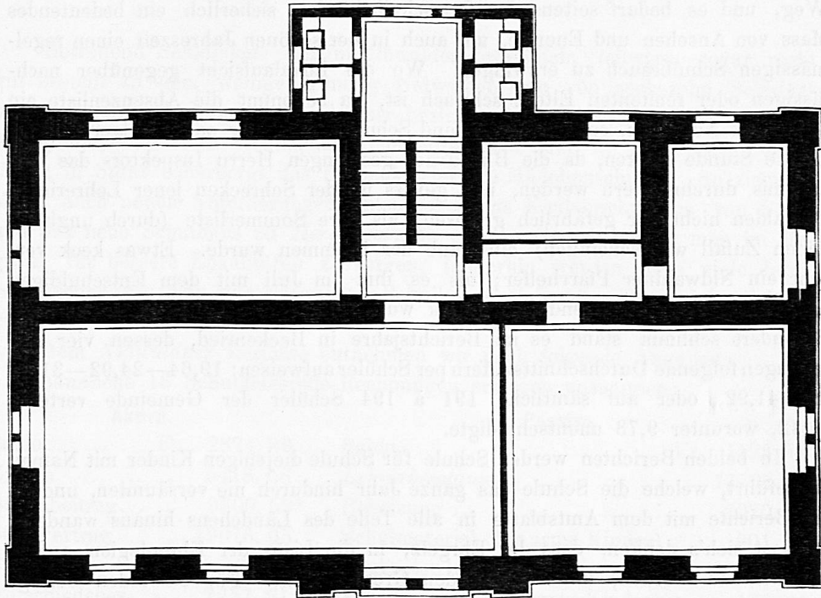
Grundriss.
