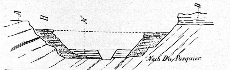
Fig. 21. Drei Glazial-Schotter; Querprofil.
