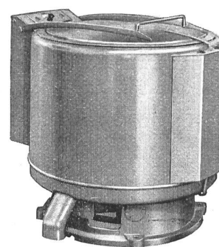
SCHULTHESS Schnellläuferzentrifuge
