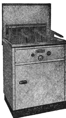
Modell Ge-Rapide Masse: 60×55×88 cm. Ölbassin: Inhalt 35 l, Anschlusswert 15 kW Fr. 2650.—
