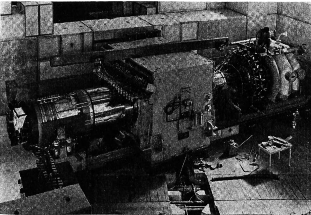
Abbildung 13 1000-l-Propankammer
