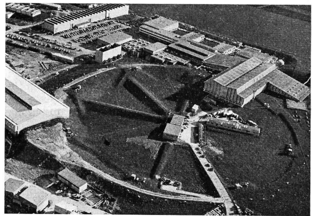
Abbildung 5 Gesamtansicht des CERN-28 GeV Proton-Synchrotrons (PS)
