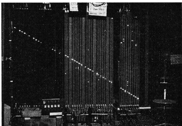
Abbildung 21 Funkenkammer
