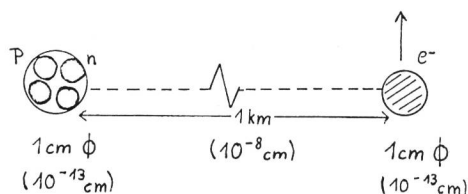
Abbildung 1 Helium-Atom
