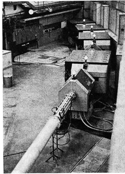
Abbildung 24 Strahlführung eines herausgelenkten Teilchenstrahls vom CERN-PS.
