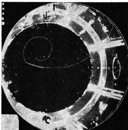
Abbildung 34 Neutrino-Reaktionen in der CERN 1000-1-Propankammer
