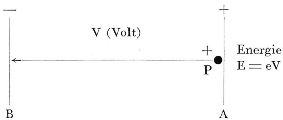
Abbildung 3 Beschleunigungsprinzip im elektrischen Feld
