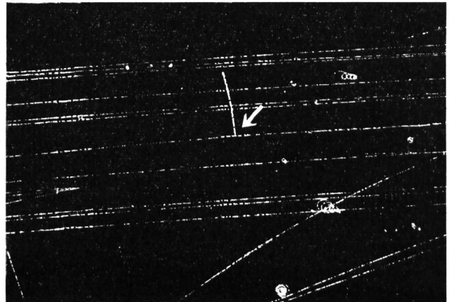
Abbildung 20 Elastische p+p -Streuung in einer Wasserstoff-Blasen-kammer. Nach der Streuung fliegen die beiden Protonen unter 90^\circ auseinander (siehe Pfeil).
