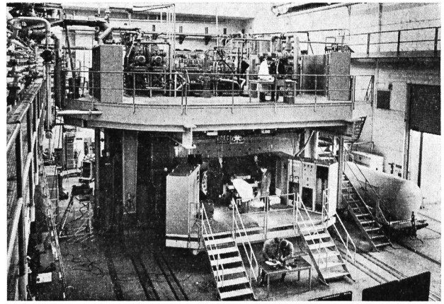
Abbildung 19 Gesamtansicht der CERN Wasserstoffkammer in Betrieb am 30 GeV Proton-Synchrotron in Genf.
