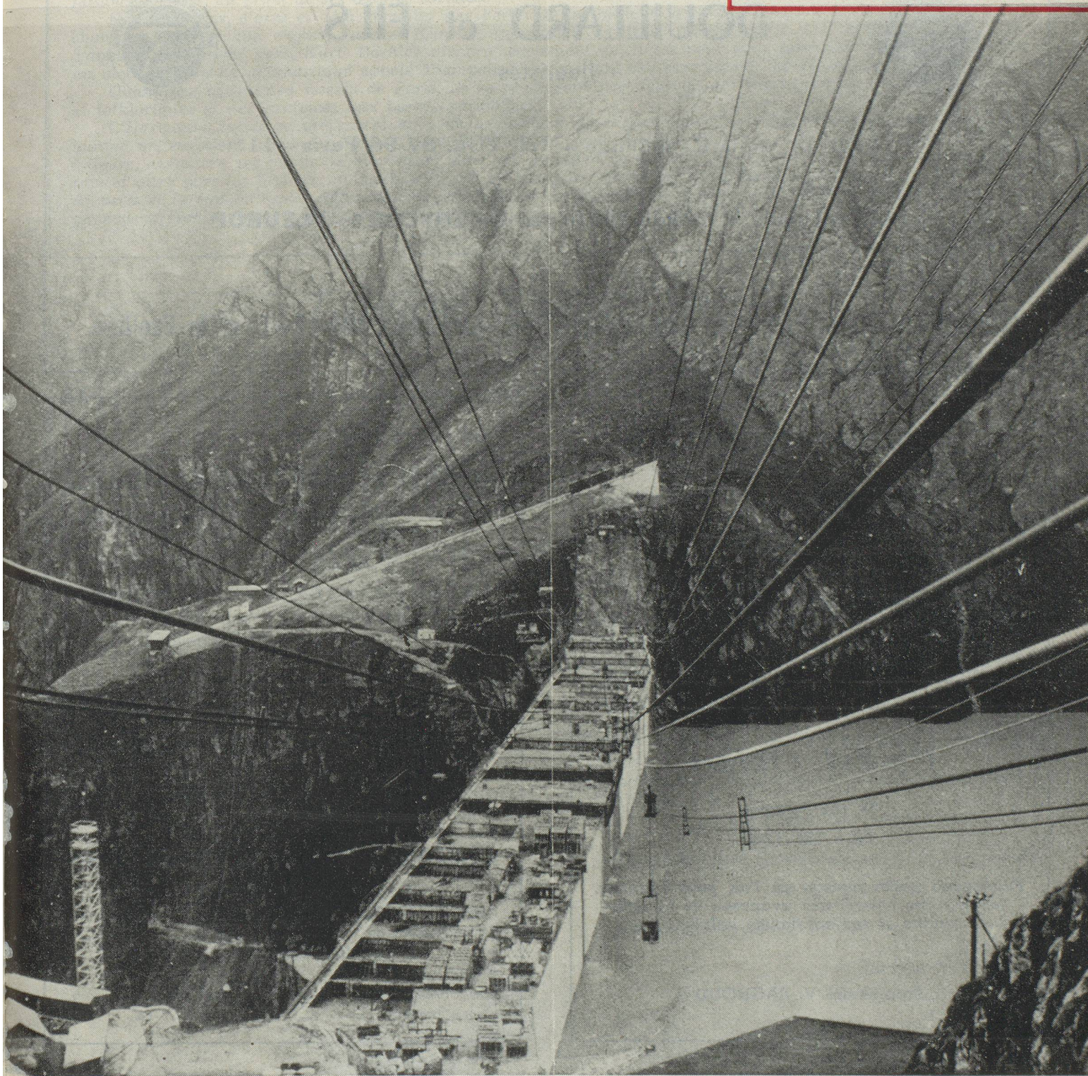
Le barrage en construction, aux deux tiers environ de sa hauteur définitive. Quatre séries de câbles gigantesques
