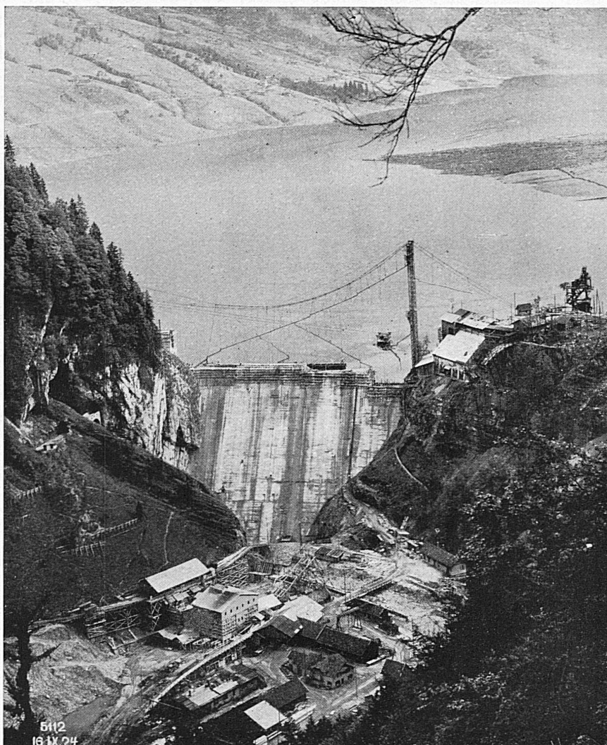
Staumauer im „Schräh“, Wäggitai, mit Installationsanlagen gemeinsam ausgeführt mit Firma Ed. Züblin & Co. A.-G., Zürich
