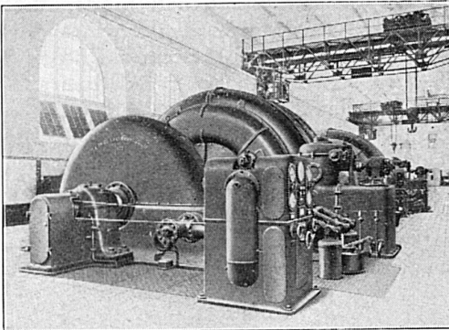
Maschinensaal im SBB-Kraftwerk Barberine, Wallis, mit vier Pelton-Turbinen à 17 000 PS Leistung
