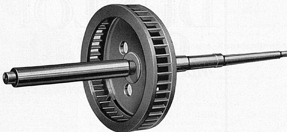
TURBINEN-SCHAUFELRAD MIT EINGEGOSSENEN P-M-G-METALL-SCHAUFELN UND GESCHMIEDETER P-M-G-METALLWELLE
