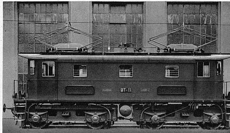
Elektrische Lokomotive der Bodensee-Toggenburgbahn
