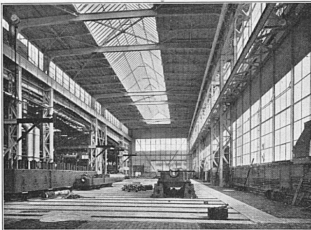
Moderne Gross-Montagehalle von 100 m Länge, 30 m Breite und 18 m Kranbahnhöhe, als Stahlskelettbau erstellt. Gewicht der Eisenkonstruktion: 613 Tonnen.
