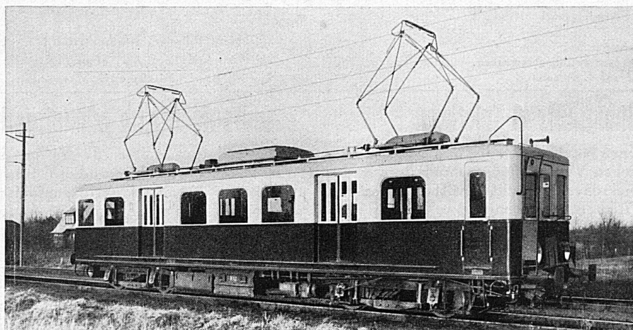
Chemin de Fer de BRUXELLES à TERVUEREN Automotrice à courant continu 1500 volts, commande à unités multiples Système SÉCHERON
