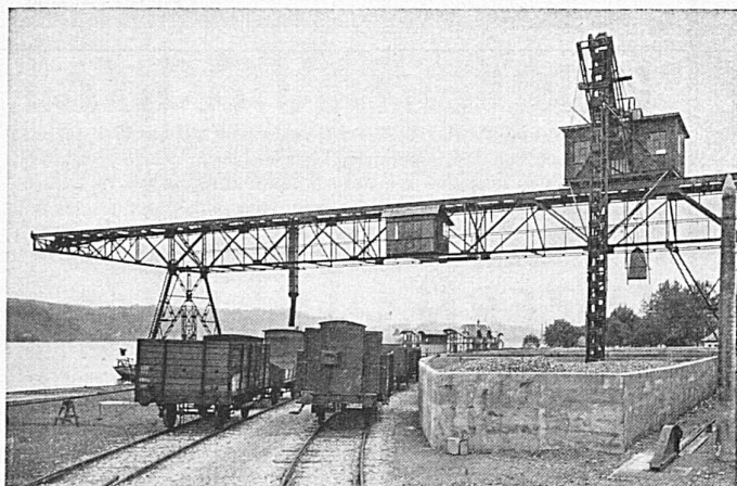
Kranbrücke einer Kies- und Sand-Verladeanlage
