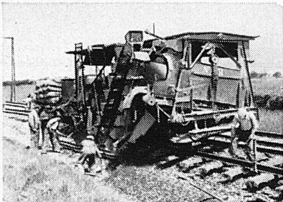
Cribleuse
