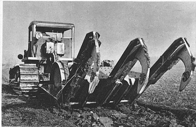
Tank - scaridefonneur. — Brevet E. G. T. 18 tonnes. — Capacité journalière de labourage 10.000 m 2 .
