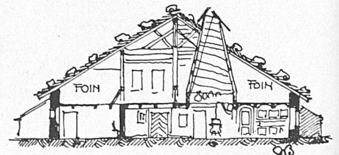
Unten: Querschnitt durch ein Jura-Haus in La Sagne. — Ci-dessous: Coupe d'une maison jurassienne située à La Sagne.
