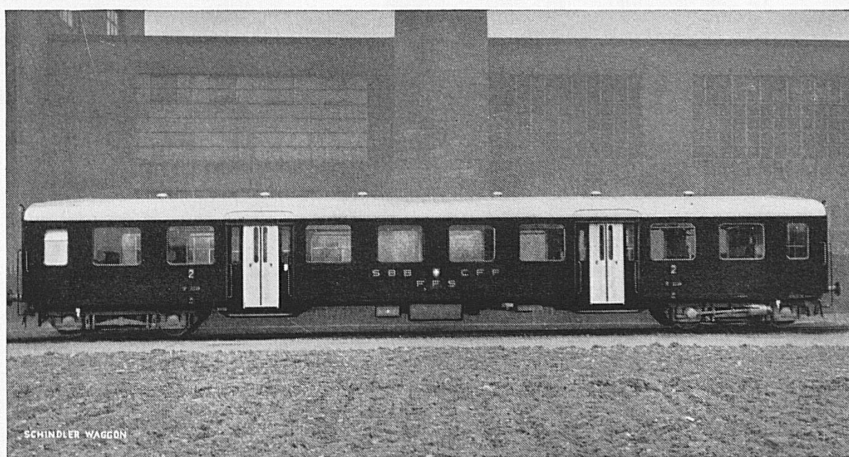
Personenwagen 2. Klasse der Schweizerischen Bundesbahnen in leichter Stahlkonstruktion, Tara 28 t
