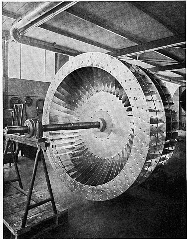
Doppel-Ventilatorrad in Aluminium für 120 000 m 3 /h
