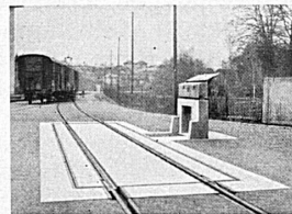
Brückenwaage für Geleise- und Straßenfahrzeuge. Wägefähigkeit 70 000 kg
