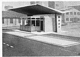
Automatische Verbund-Brückenwaage für Straßenfahrzeuge. Wägefähigkeit je 30 000 kg
